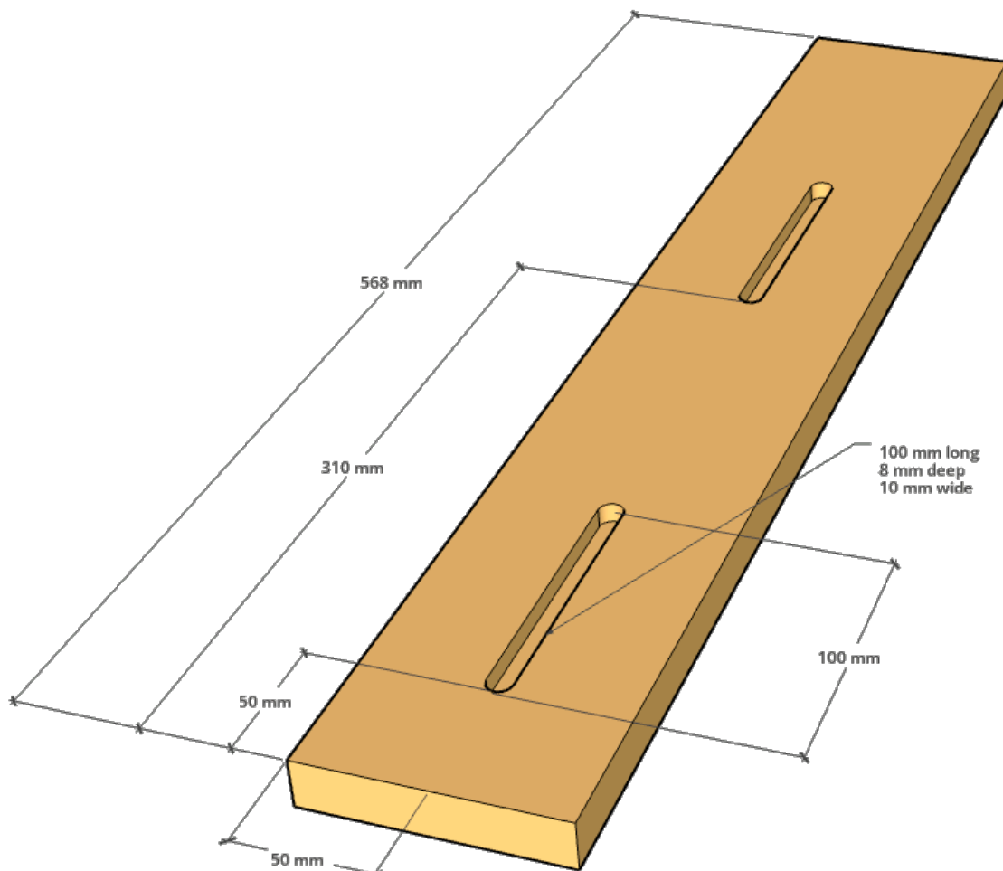
Figur 106 Bräde med slitsar
