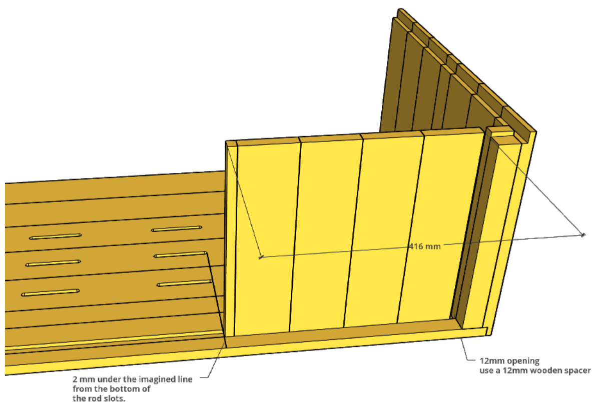
Figur 120 Lägg till fler innerväggstavlor
