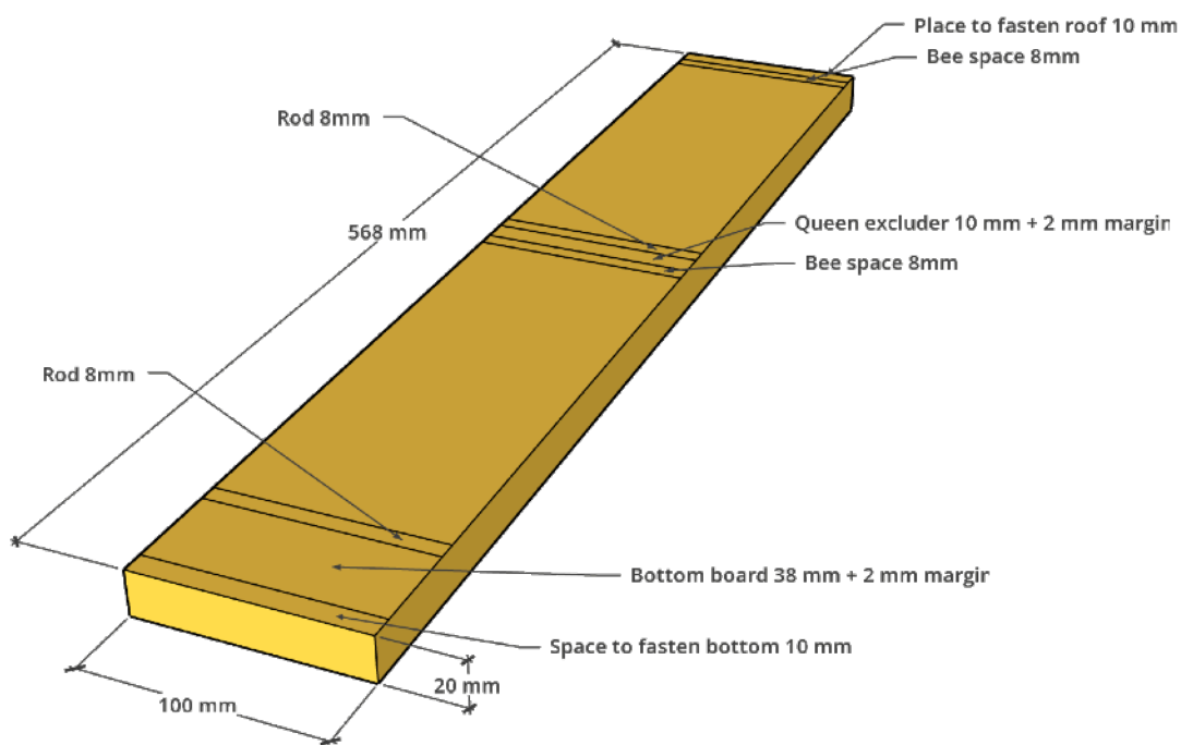
Figur 104 Beräkna sidobrädan
