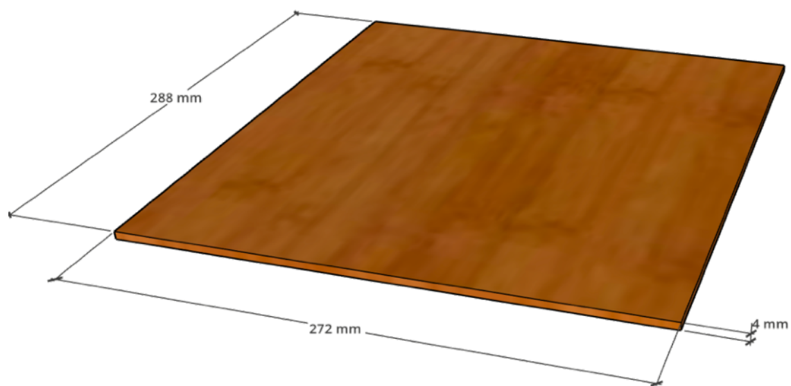
Figur 111 Plywood för spegel på dörren
