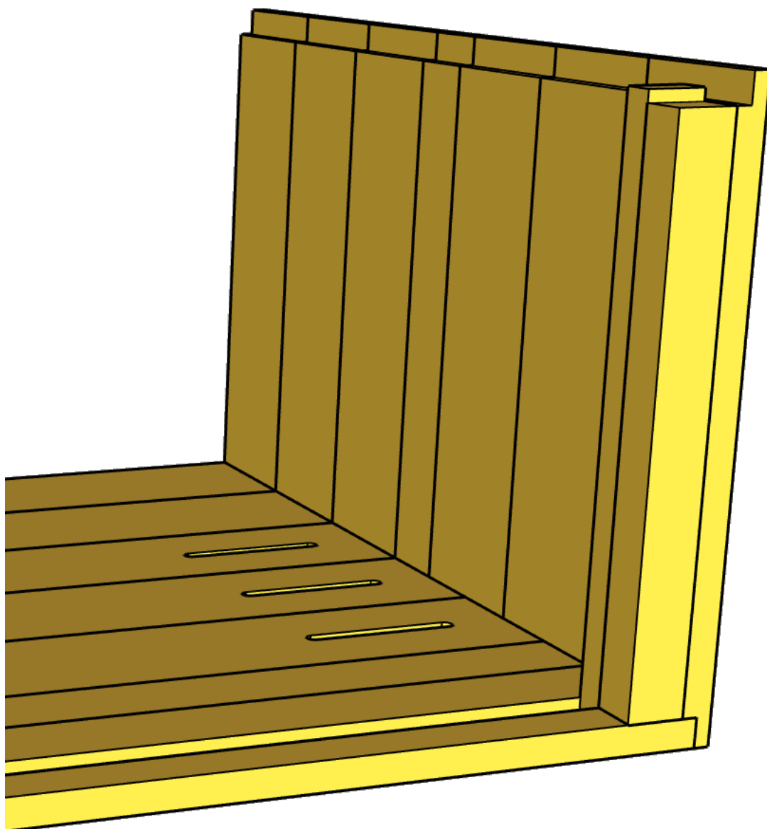
Figur 119 Mellan bräddor för entrén.
