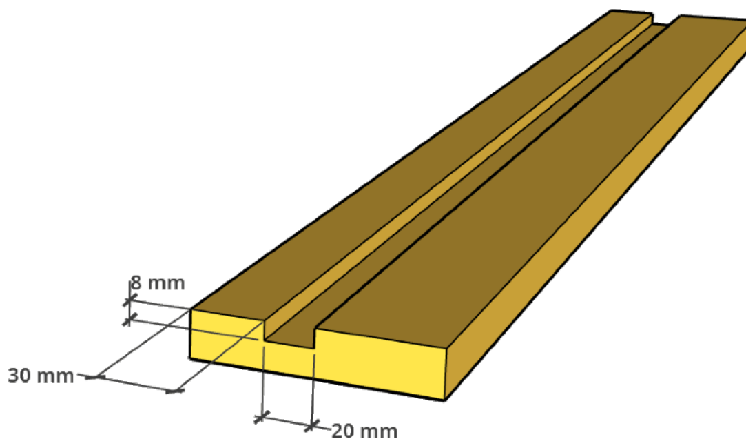
Figur 105 Första sidobrädan framåt
