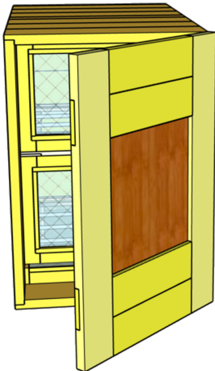
Figur 132 Färdig bikupa
