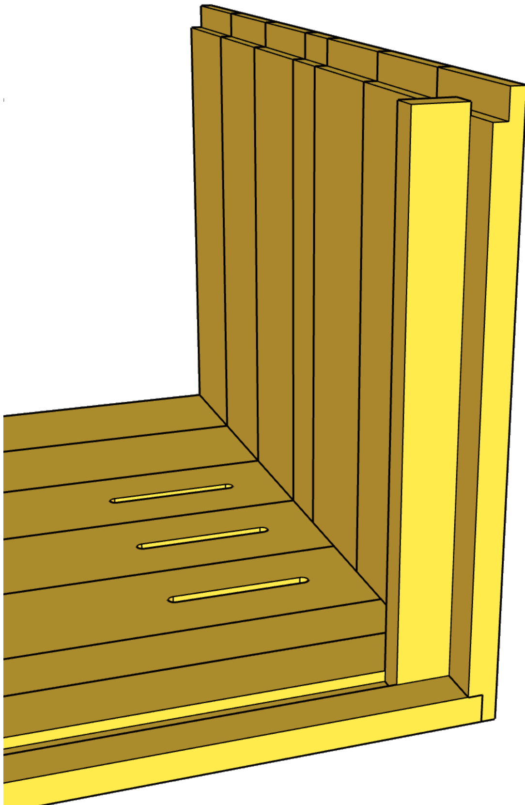
Figur 118 Första innerväggstavlan
